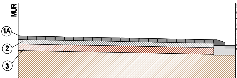
SECCIÓ PAVIMENT VORERA
