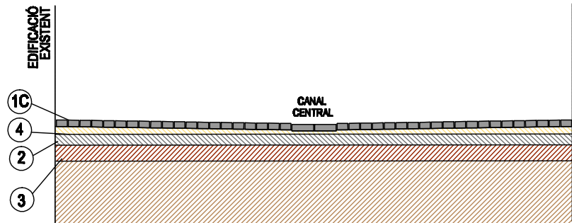
SECCIÓ PAVIMENT POSTERIOR I LATERAL ARXIU
