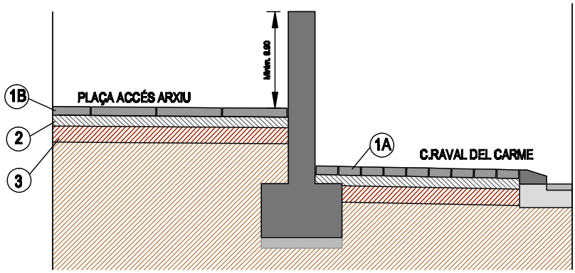
SECCIÓ PEL MUR DE CONTENCIÓ
