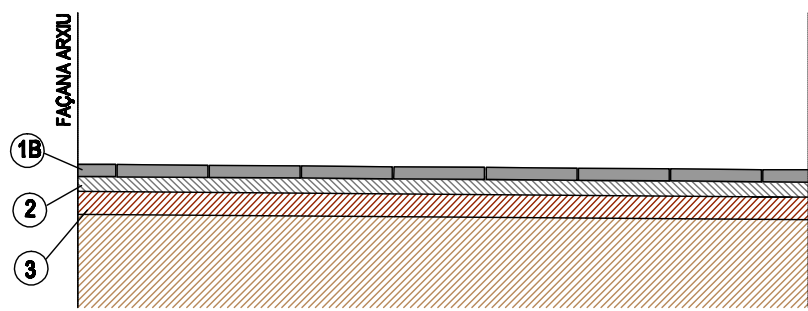
SECCIÓ PAVIMENT PLAÇA ACCÉS ARXIU
